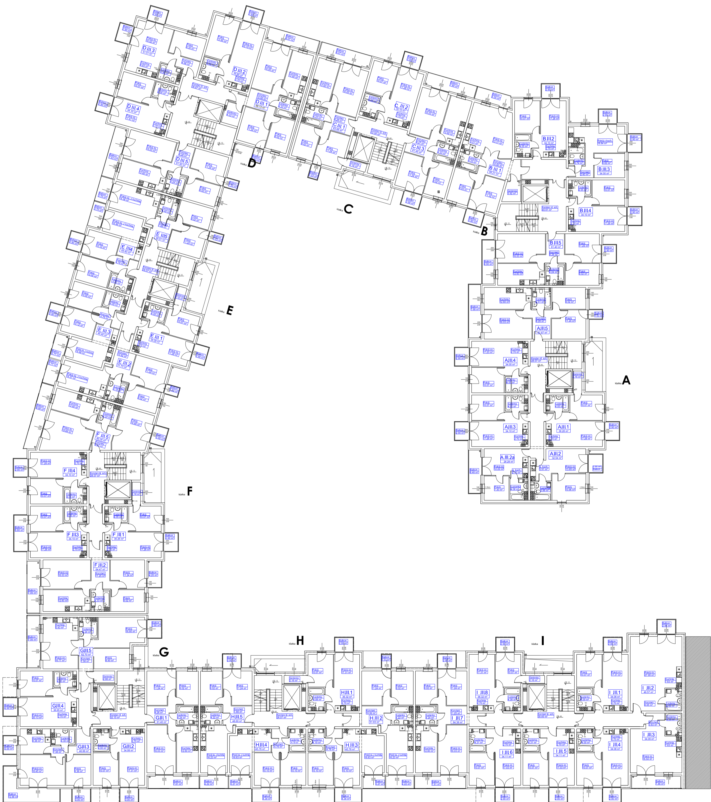
Rzut kondygnacji III 1:200
